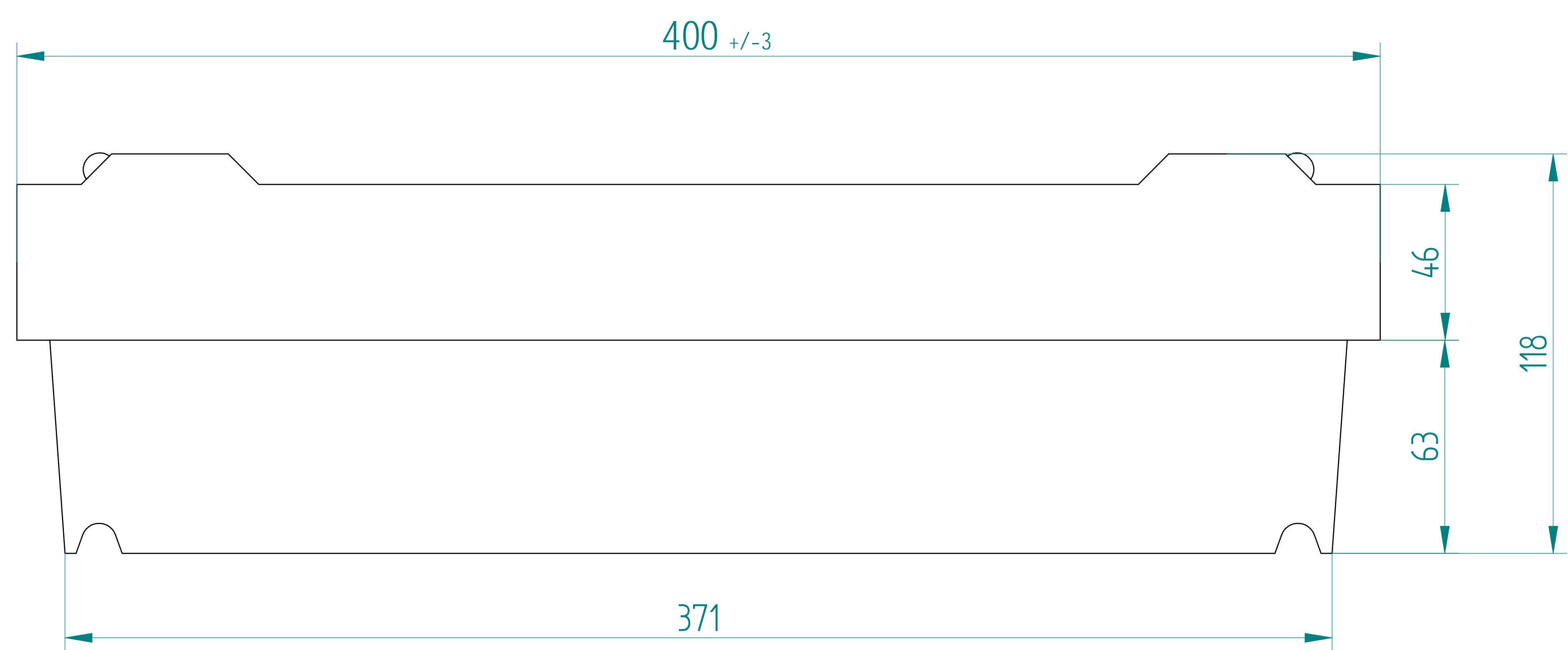
SECTION A-A
