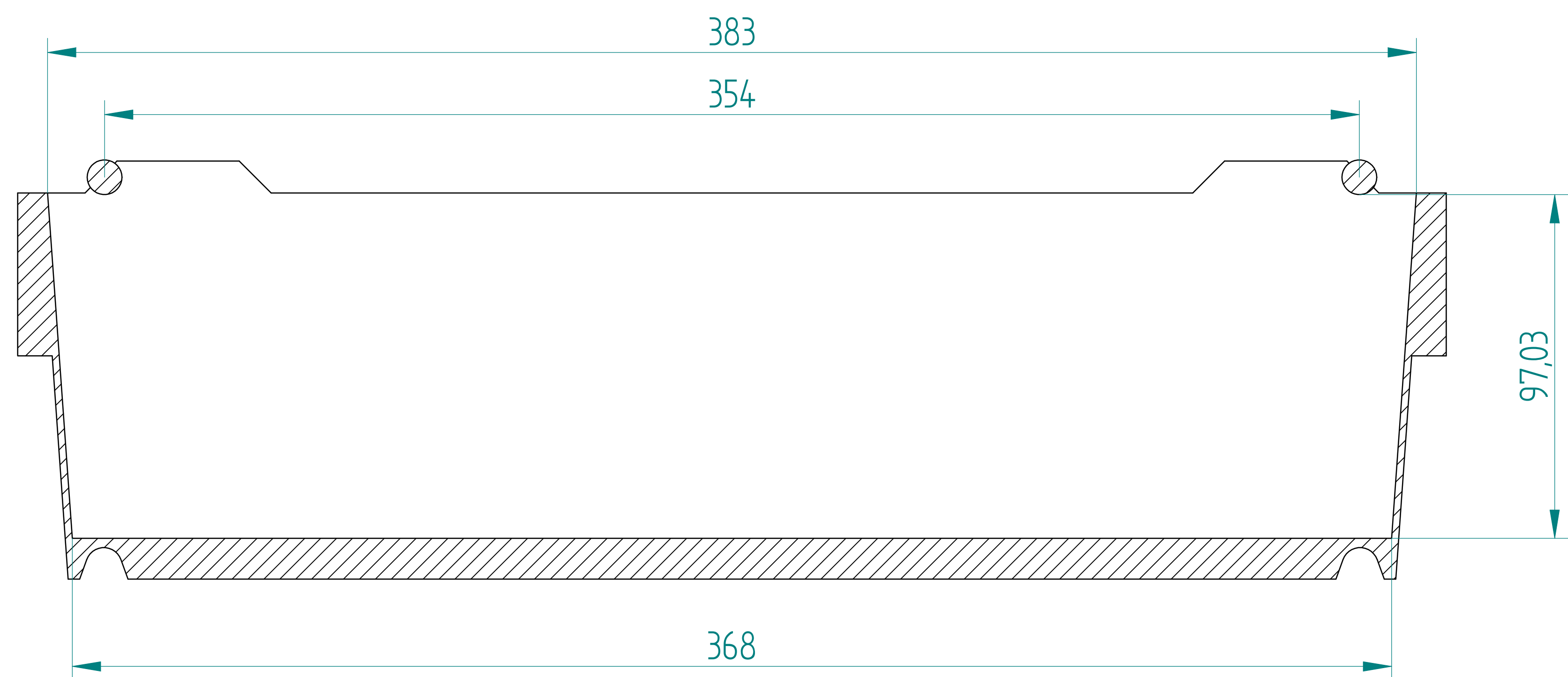
SECTION A-A
